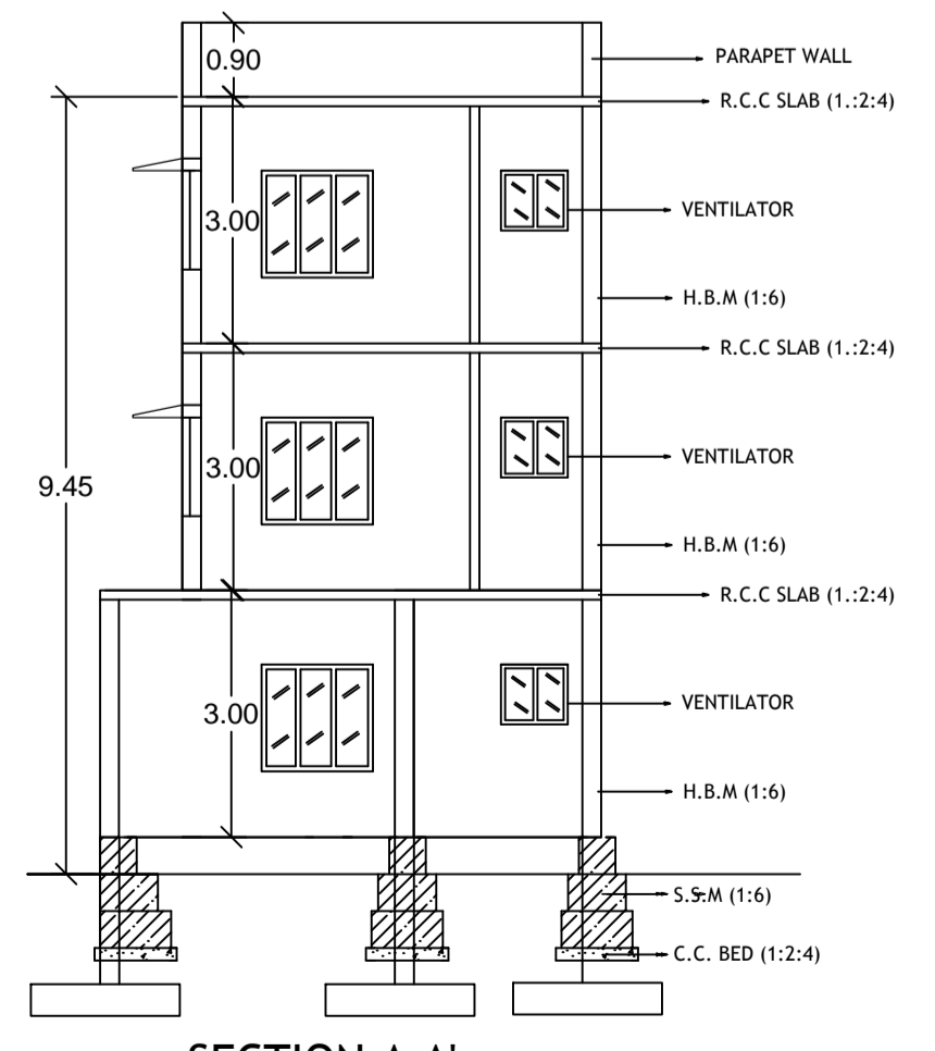
SECTION A-A
